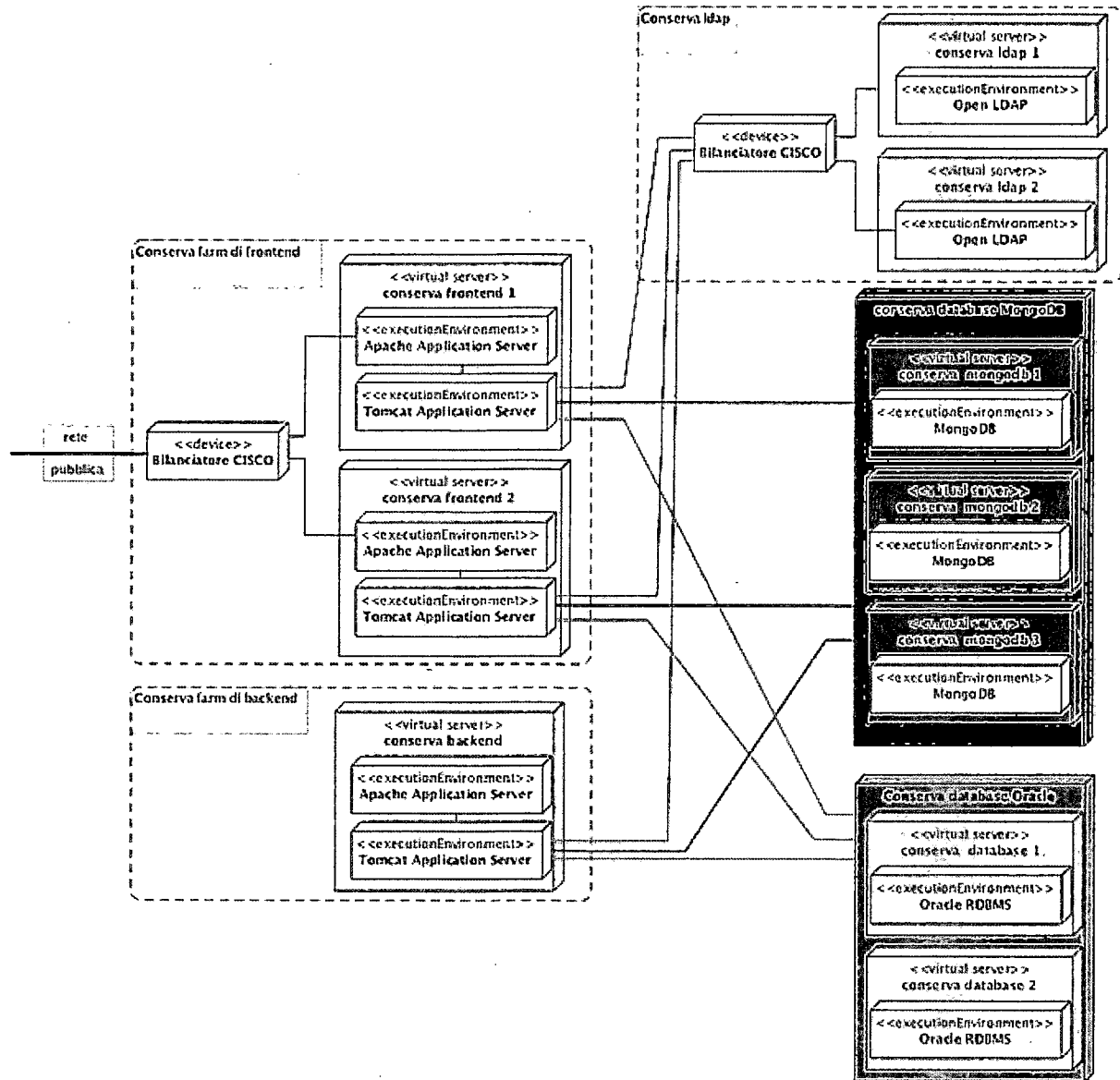
Figura 4 - Distribuzione componenti di Conserva
