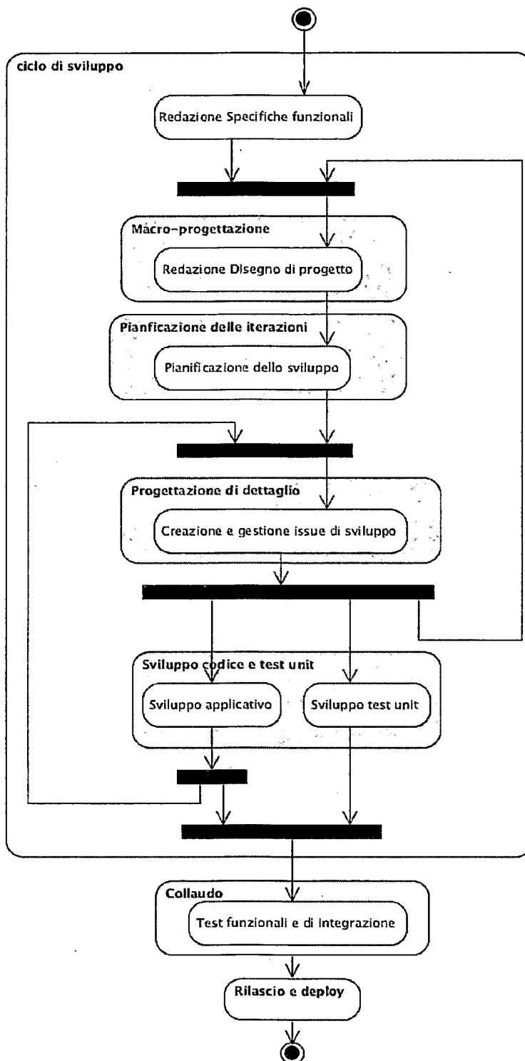
Figura 9 - Fasi di produzione e rilascio del software
