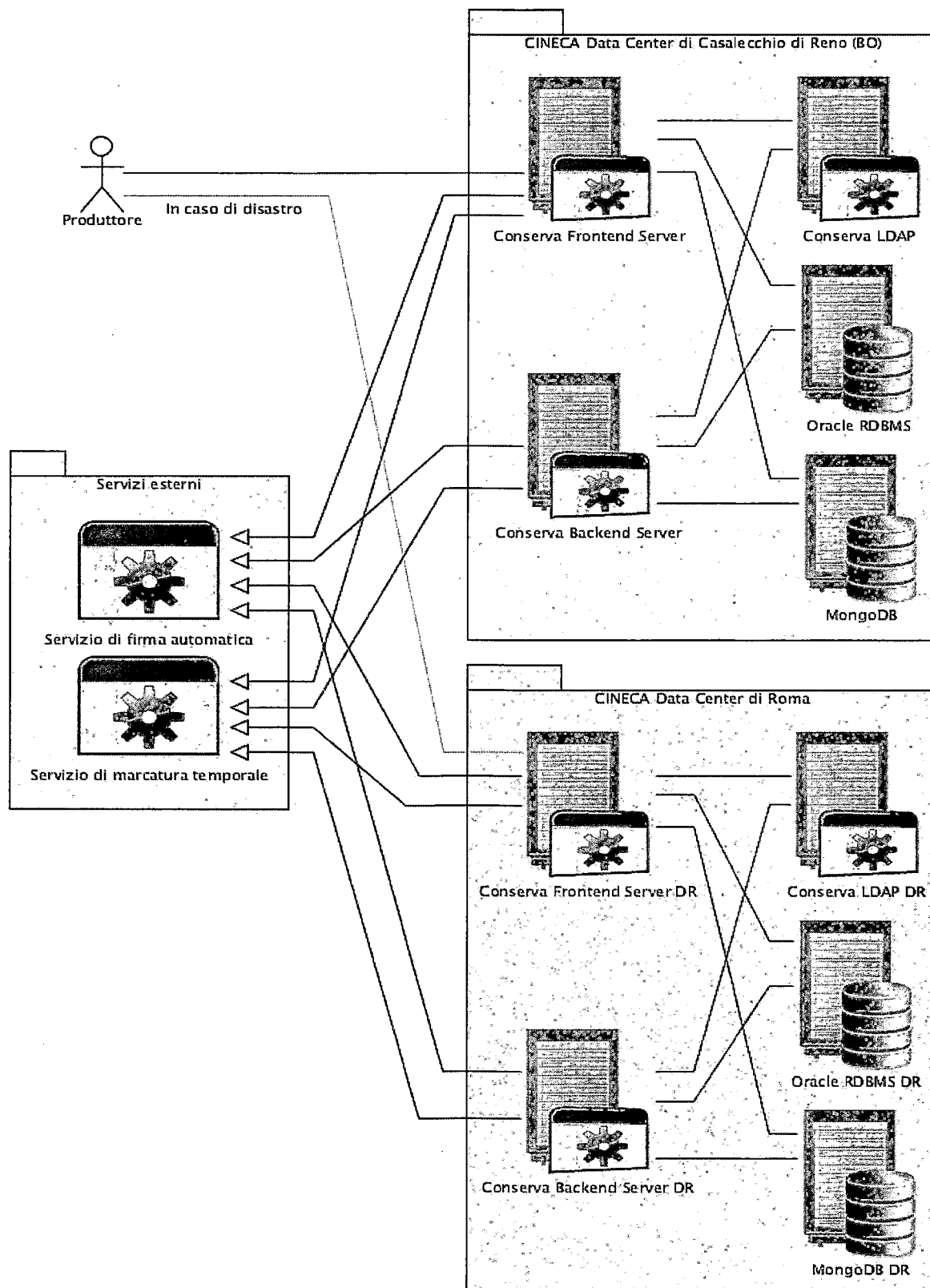
Figura 5 - Distribuzione topologica delle componenti fisiche di Conserva
